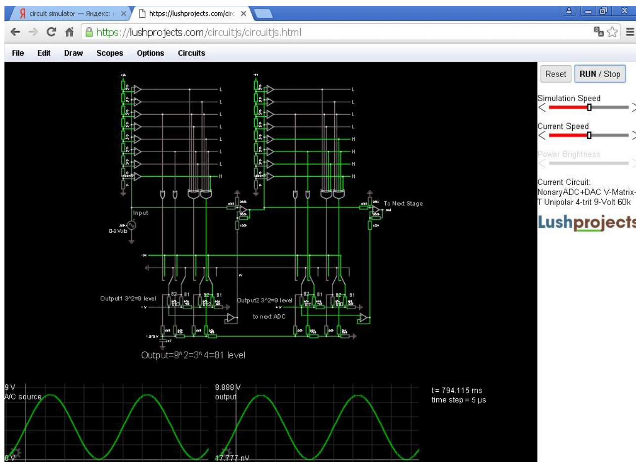
Рис.1. Снимок модели девятиричного АЦП последовательного приближения с троичным ЦАПом на резисторных матрицах напряжения 3R-4R(терминатор 6R) с аналоговыми переключателями, однополярного, 2-х нонитного (4-х тритного), в онлайн HTML5-версии симулятора электронных схем Circuit Simulator.
