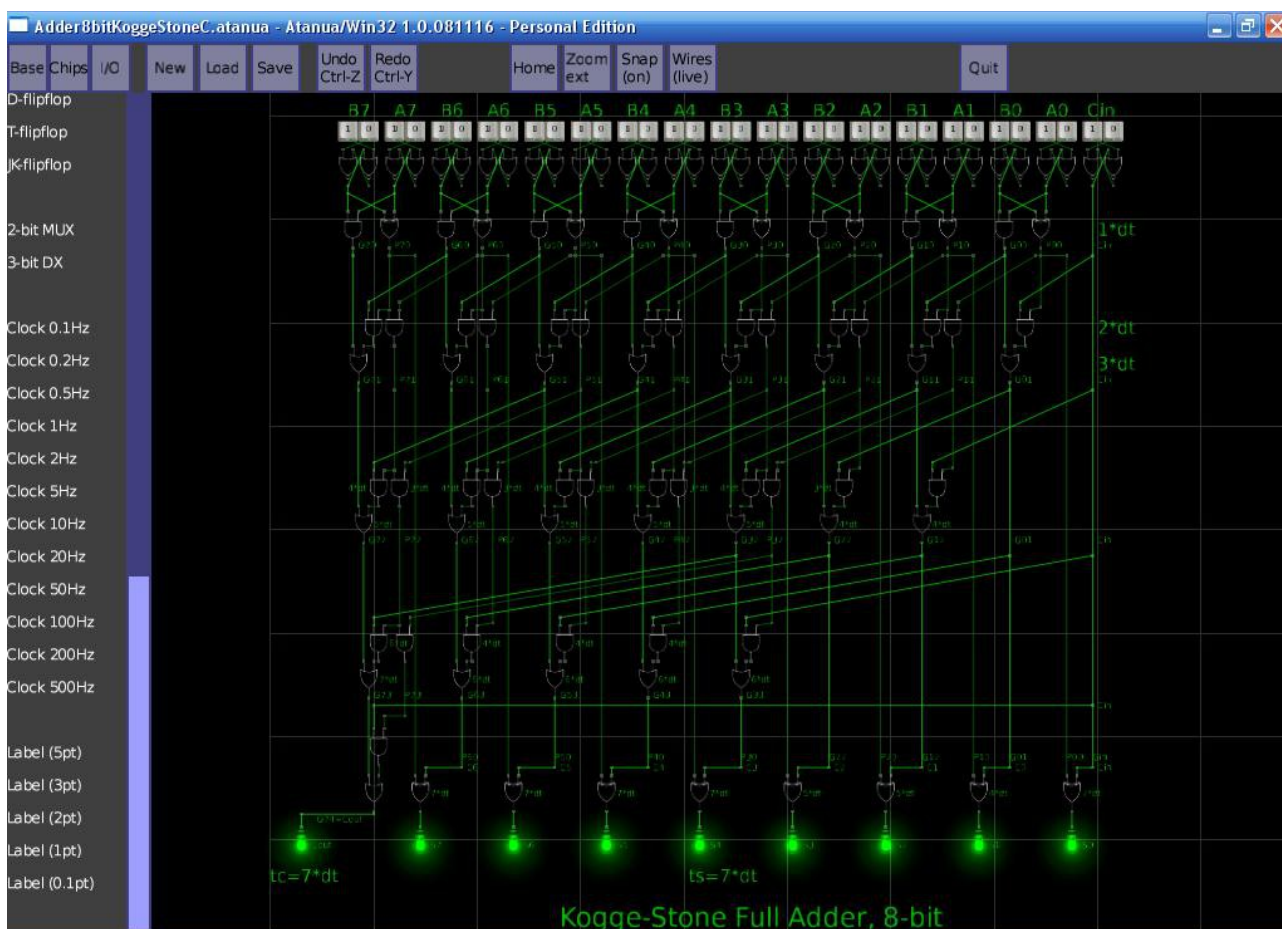
Рис.1. Снимок модели 8-ми битного (однobaйтного, 256-тиричного) полного сумматора Когге-Стоуна с битом Cin в логическом симуляторе Atanua/Win32 1.0.081116 - Personal Edition .
