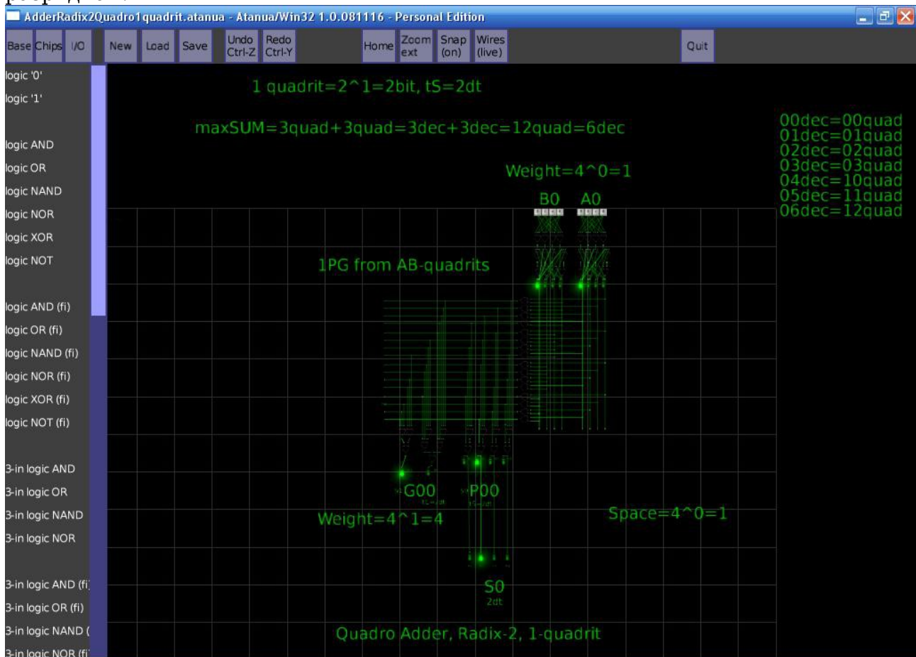
Рис.2. Снимок модели четверичного сумматора, Radix-2, 1-но квадратного, в логическом симуляторе Atanua/Win32 1.0.081116 - Personal Edition .
