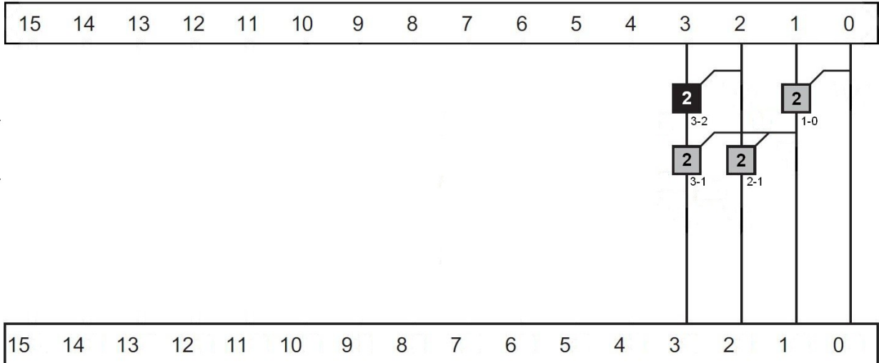
Рис.1. Граф генератора переносов двоичного сумматора Скланского, Radix-2, 4-х разрядного (используются только двухвходовые операторы 2G (Gray2) Cell (без вычисления оператора 2P) и 2PG (Black2) Cell).
