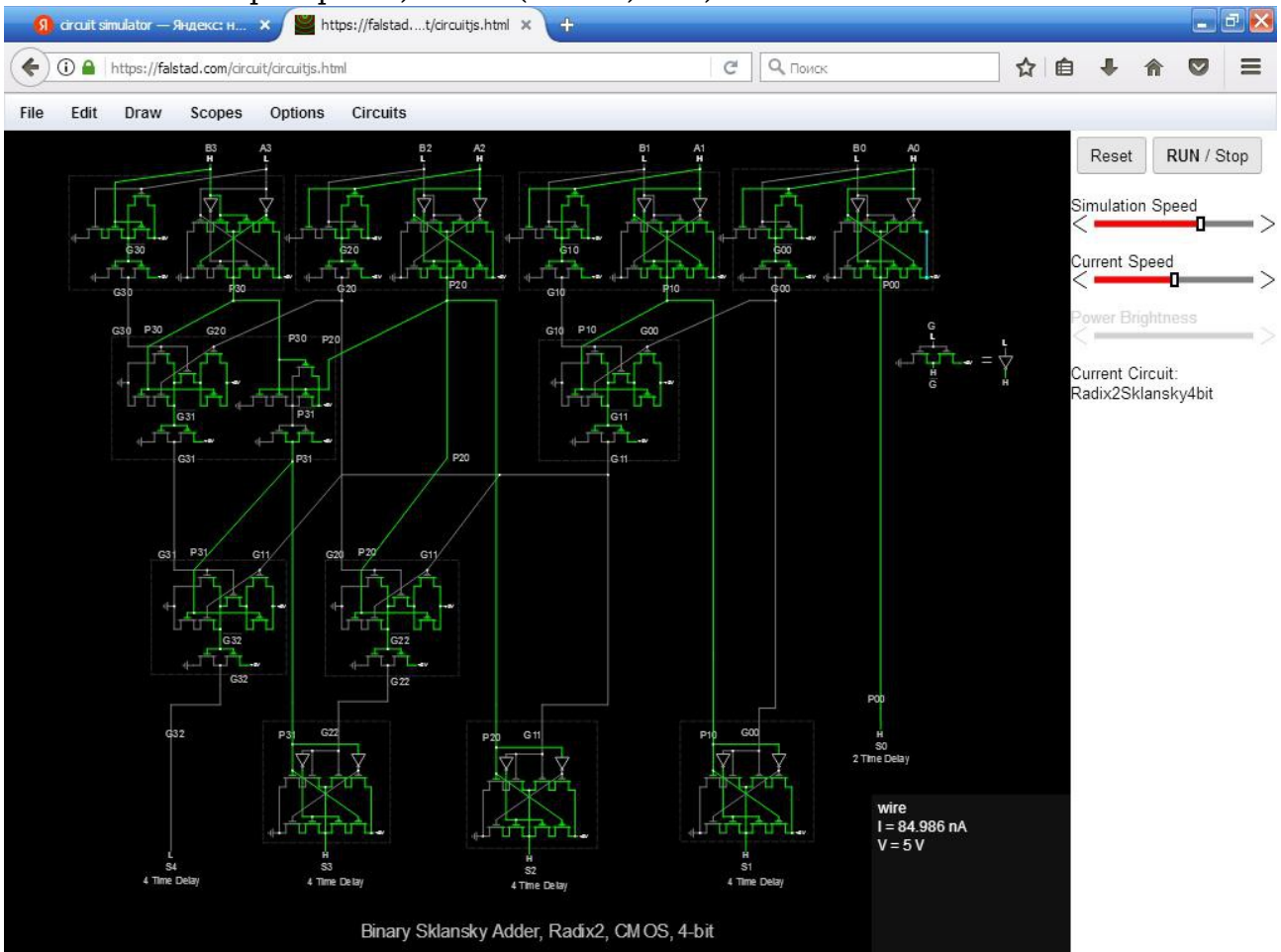
Рис.2. Снимок модели двоичного сумматора Скланского, Radix-2, CMOS версия, 4-х битного (полубайтного) в Circuit Simulator'e.
