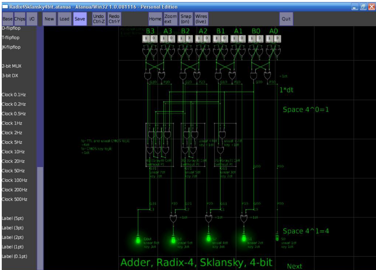
Рис.2. Снимок модели сумматора Скланского, Radix-4, 4-х битного (полубайтного, 16-тиричного, гексадецичного) в логическом симуляторе Atanua/Win32 1.0.081116 - Personal Edition .
