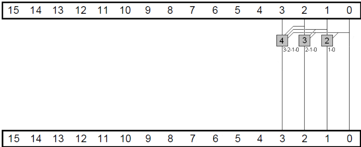
Рис.1. Блок-схема генератора переносов сумматора Скланского, Radix-4, 4-х битного (используются двух, трёх и четырёх входные (аргументные) операторы (функции) 2G, 3G и 4G (Gray2, Gray3 и Gray4) (без вычисления функций 2P, 3P и 4P)). Порядок подключения входов имеет значение.
