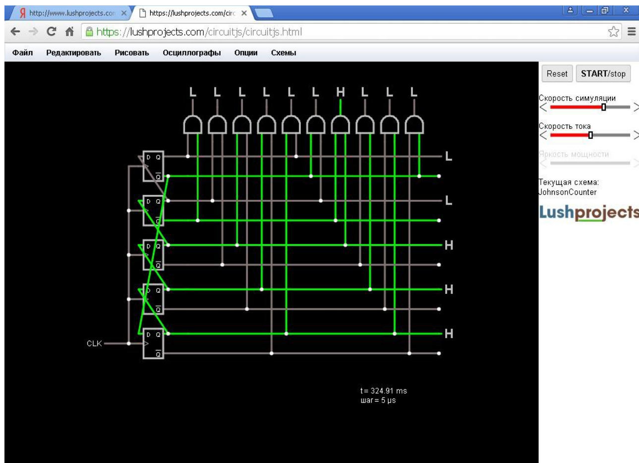
Рис.1. Снимок модели счётчика Джонсона с дешифратором в онлайн версии логического симулятора Circuit Simulator.
