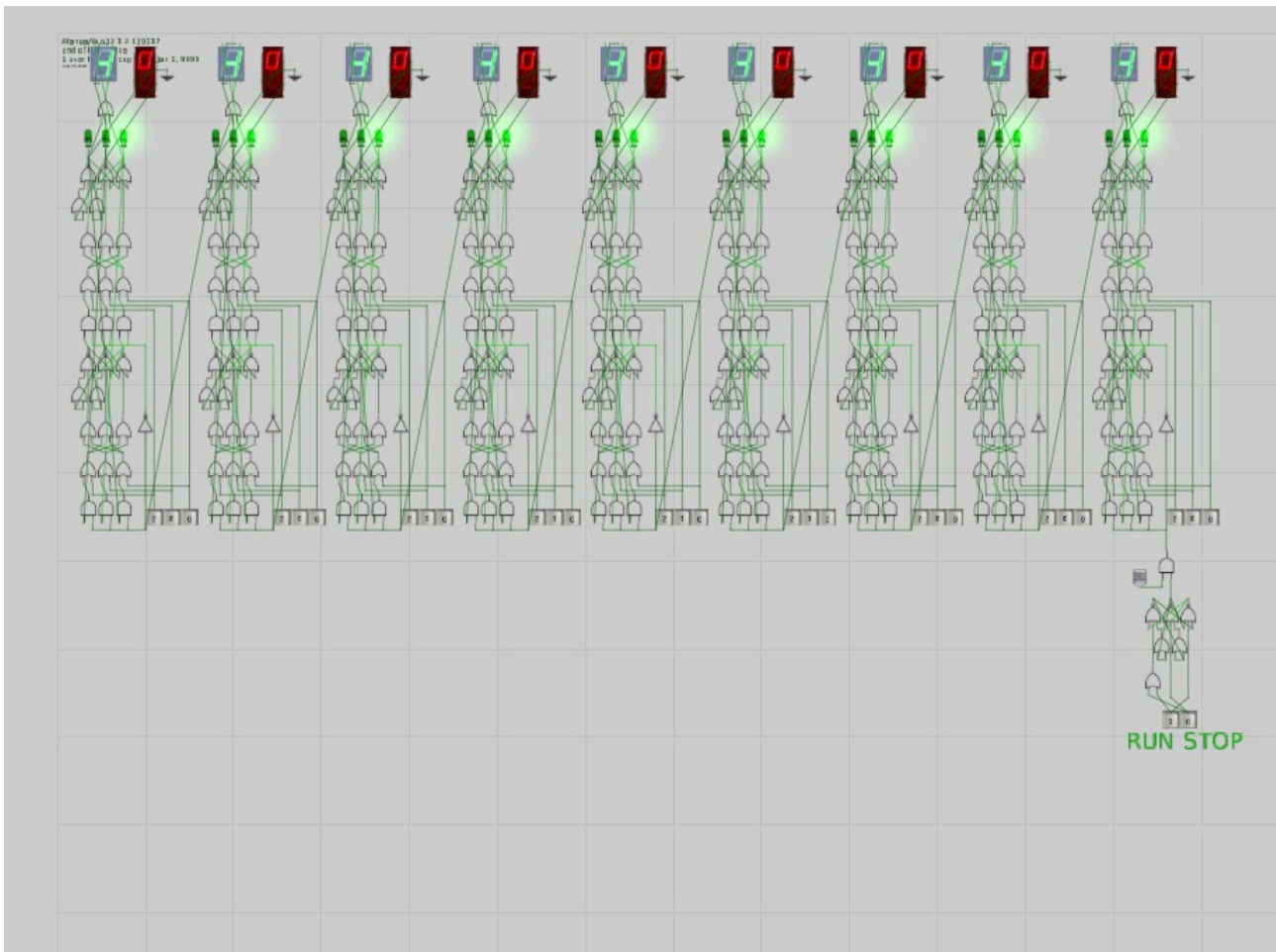
Рис.1. Снимок модели троичного несимметрично-симметричного трёхбитного счётчика адреса команд, 9-ти тритного, в логическом симуляторе Atanua/Win32 1.2.130617.
