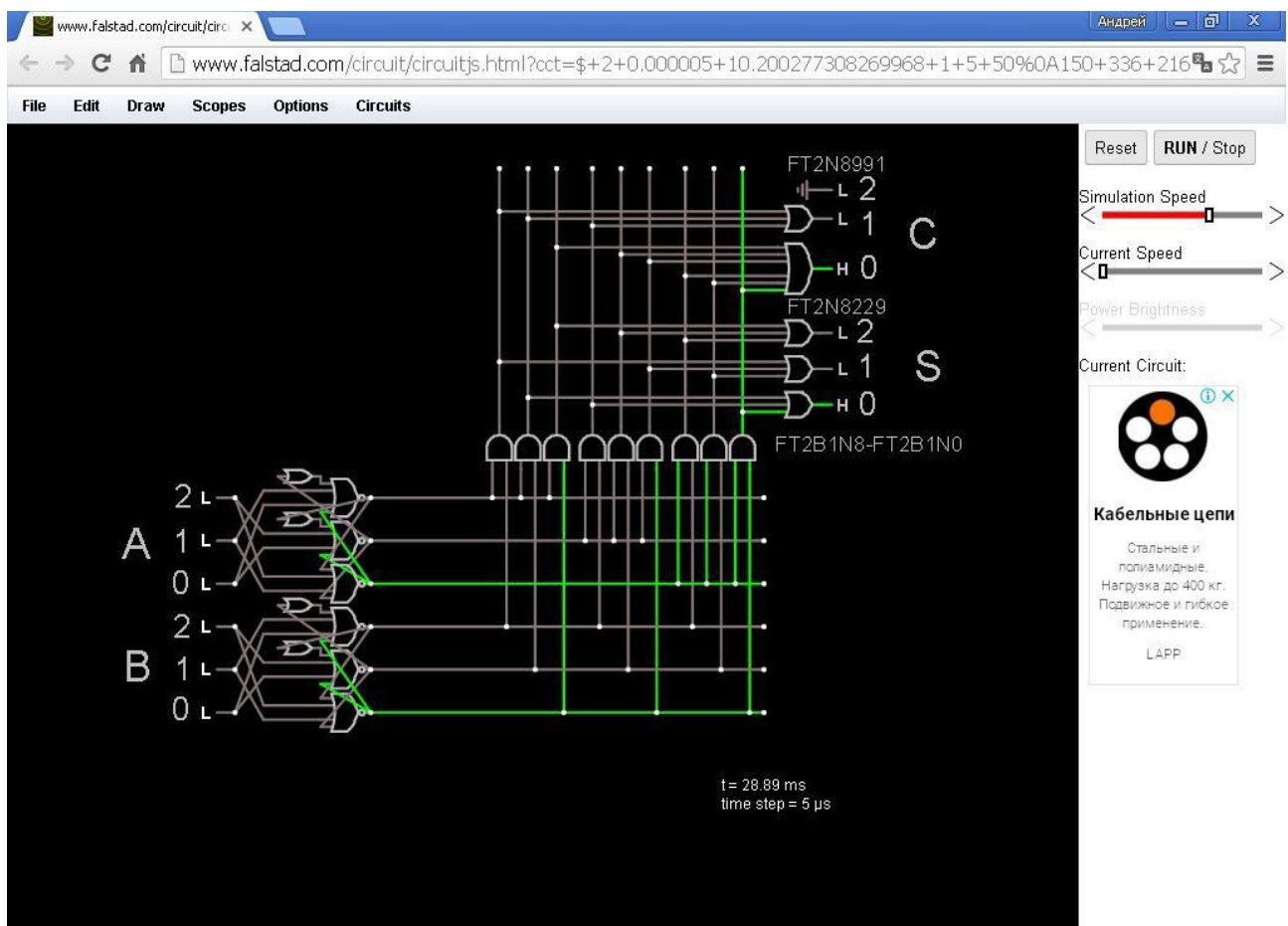
Рис.1. Снимок модели троичного полусумматора, несимметричного, в трёхбитной (в «трёхпроводной») системе троичных логических элементов в онлайн HTML5-версии симулятора электронных схем Circuit Simulator.
