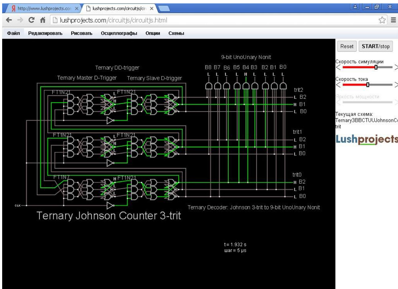
Рис.1. Снимок модели троичного 3-х тритного кольцевого регистра сдвига (троичного счётчика Джонсона) на двухступенчатых D-триггерах (DD-триггерах) с дешифратором в онлайн версии симулятора электронных схем Circuit Simulator.
