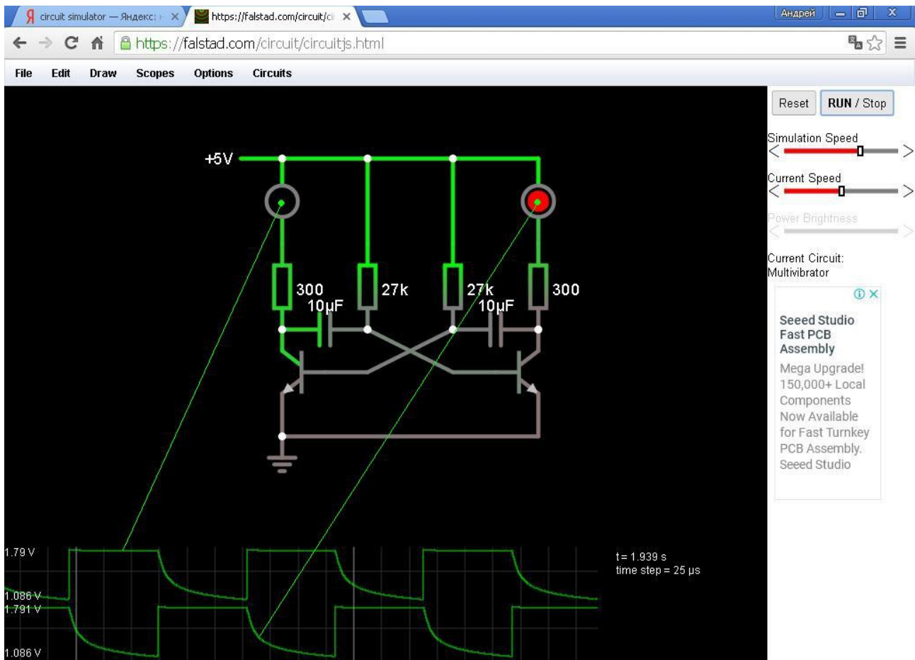
Рис.1. Снимок модели мультивибратора со светодиодами в онлайн HTML5-версии симулятора электронных схем Circuit Simulator.
