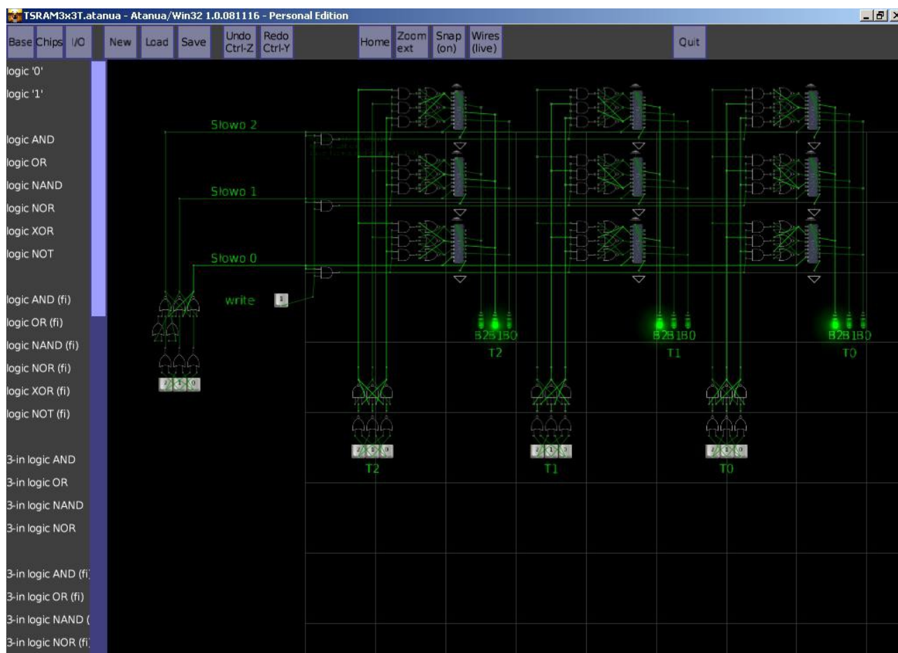
Рис.1. Снимок модели модуля троичной трёхбитной (3В ВСТ) SRAM 3x3T=9 Тритов 3xNOR3 в симуляторе логических схем Atanua/Win32 1.0.081116 - Personal Edition.
