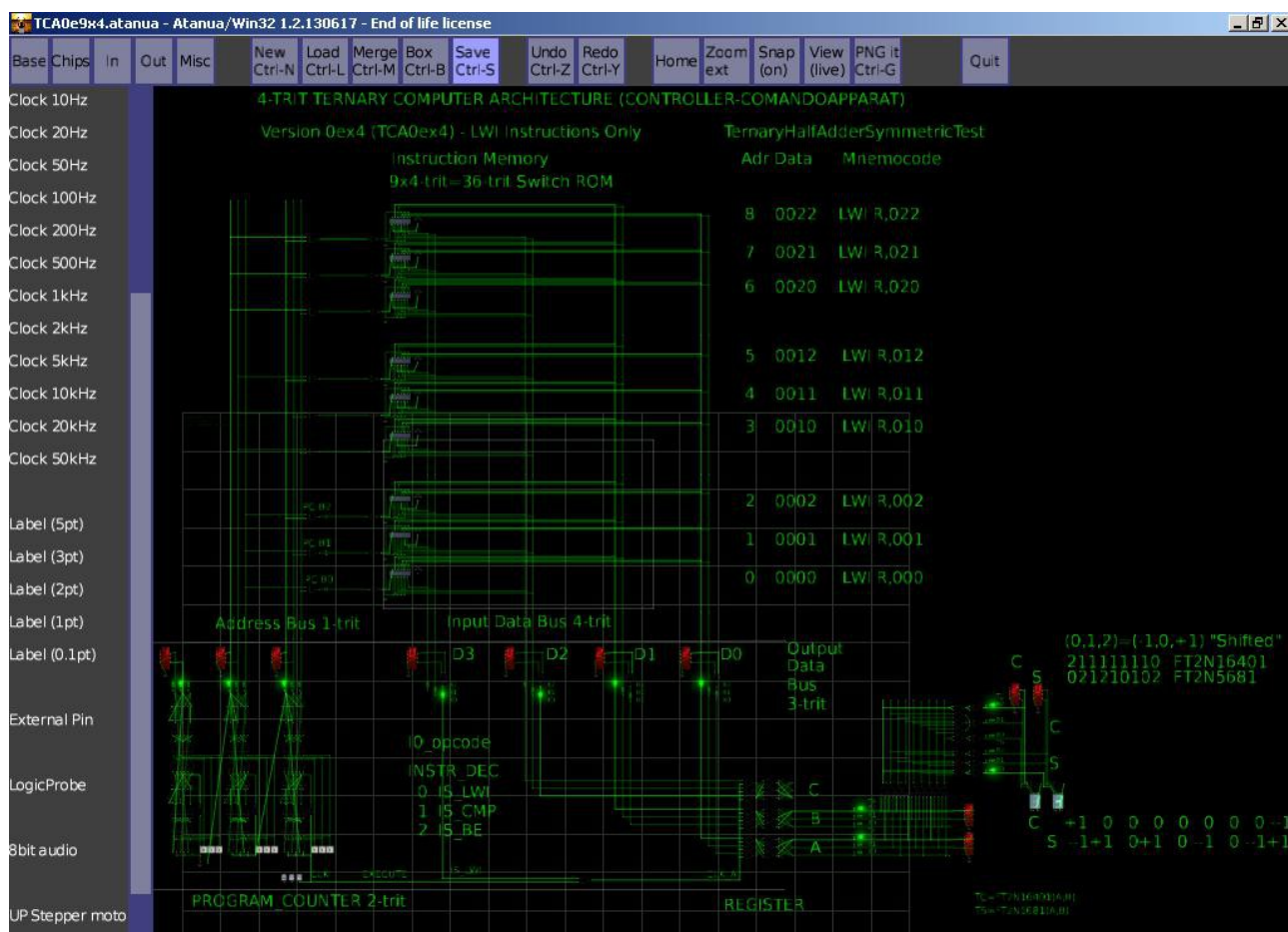
Рис.1. Снимок модели контроллерного стенда для проверки и изучения троичного симметричного трёхбитного одноединичного полусумматора «Shifted» в симуляторе логических схем Atanua/Win32 1.2.130617.
